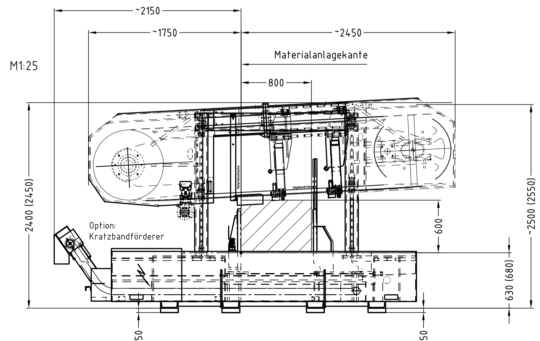
Ansicht X
